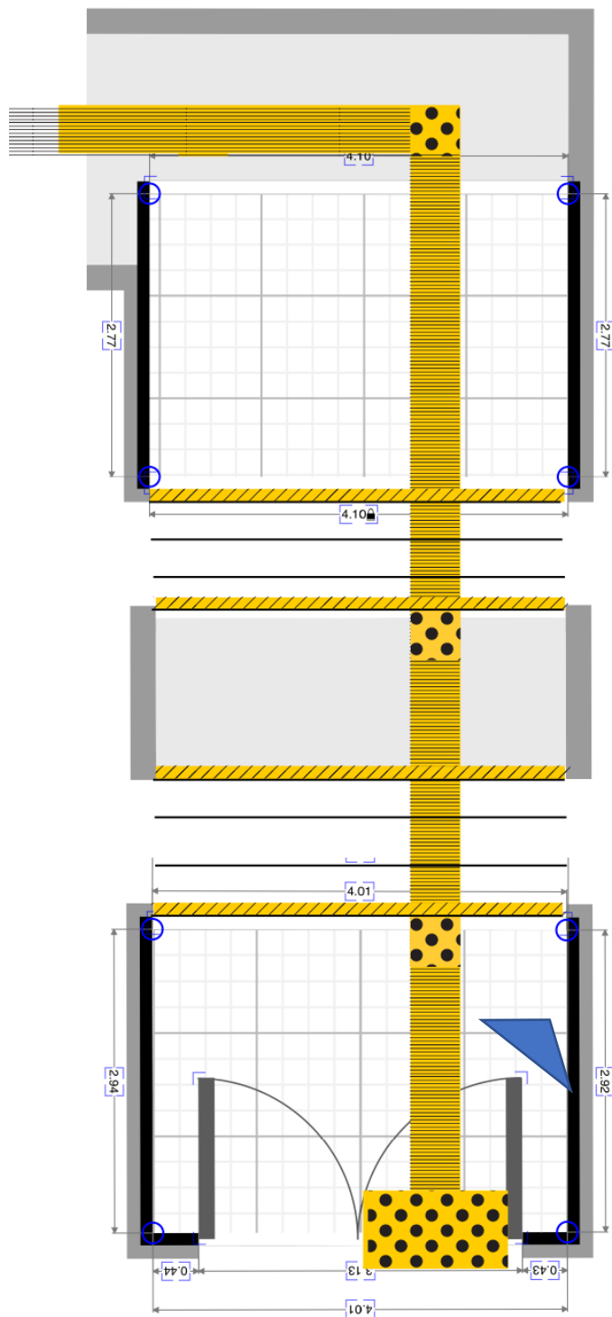
Tlocrt 2. Taktilna staza u ulazu
