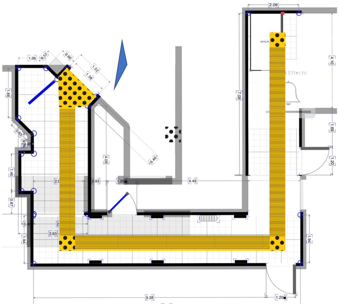
Tlocrt 3. Taktilna staza u honicima 1,2,3
